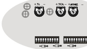
Scheda base del motore "A" "A" Motor main board Carte de base du moteur "A" Basiskarte vom Motor "A" Tarjeta base del motor «A»
