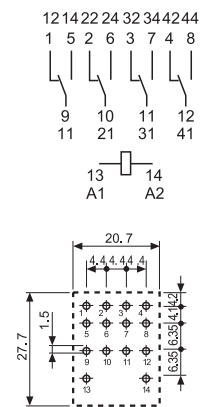
Vue coté cuivre
