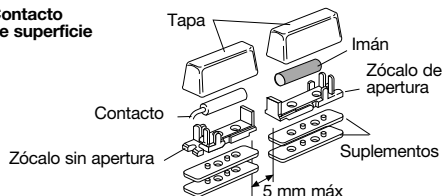
Contacto de superficie atornillado
