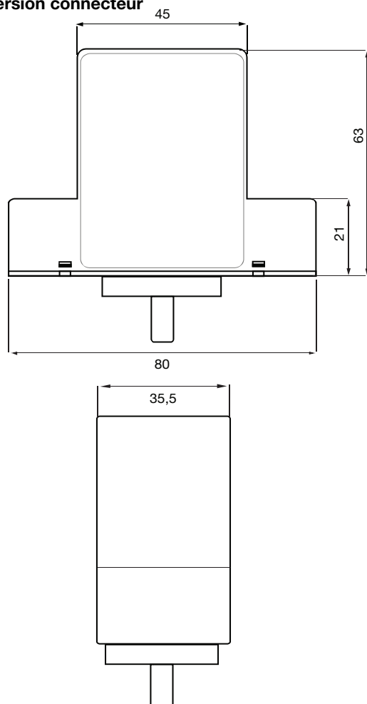
Version connecteur
